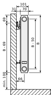
Compact, typ 21s z zawieszaniami ściennymi SSMS, widok z boku
