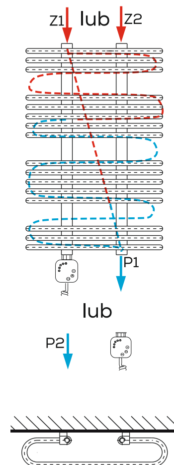
PODŁĄCZENIE KRZYŻOWE
