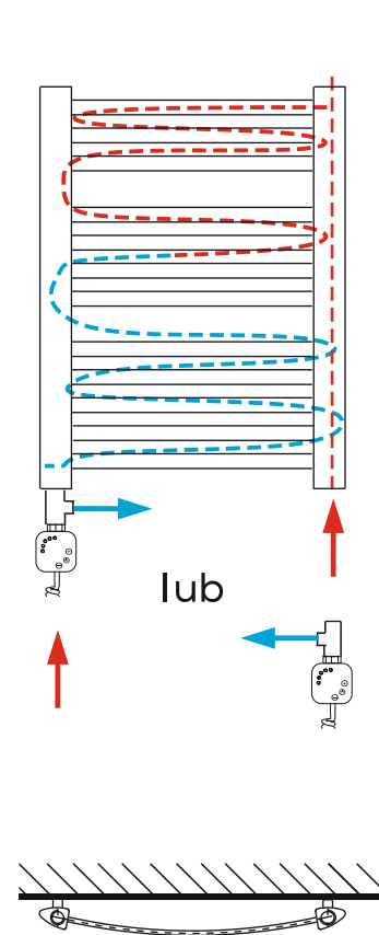
WODNO-ELEKTRYCZNY OD DOŁU W KOLEKTORACH
