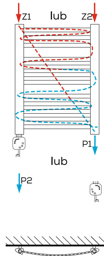
WODNO-ELEKTRYCZNY PODŁĄCZENIE KRZYŻOWE
