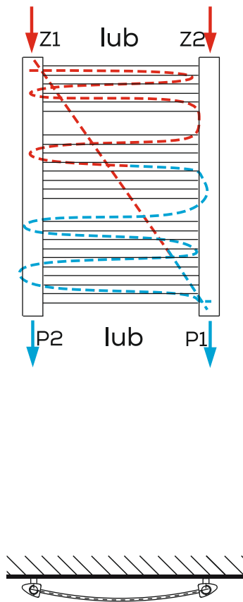
PODŁĄCZENIE KRZYŻOWE
