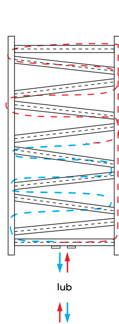
PODŁĄCZENIE DOLNE CENTRALNE
