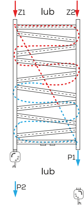
WODNO-ELEKTRYCZNY PODŁĄCZENIE KRZYŻOWE
