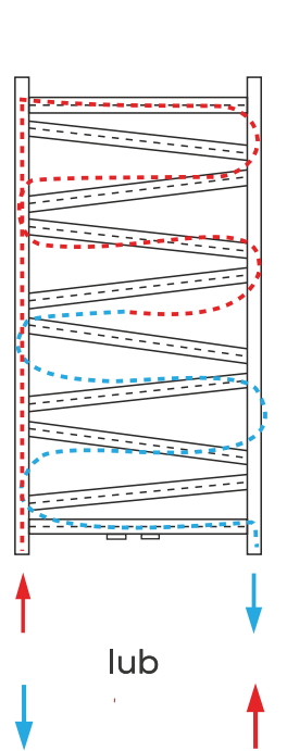
PODŁĄCZENIE OD DOŁU W KOLEKTORACH
