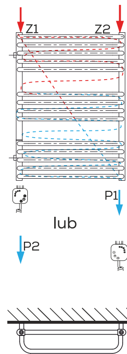
WODNO- ELEKTRYCZNY PODŁĄCZENIE KRZYŻOWE
