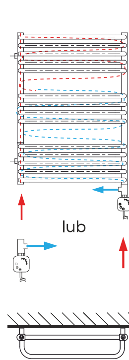
WODNO- ELEKTRYCZNY OD DOŁU W KOLEKTORACH
